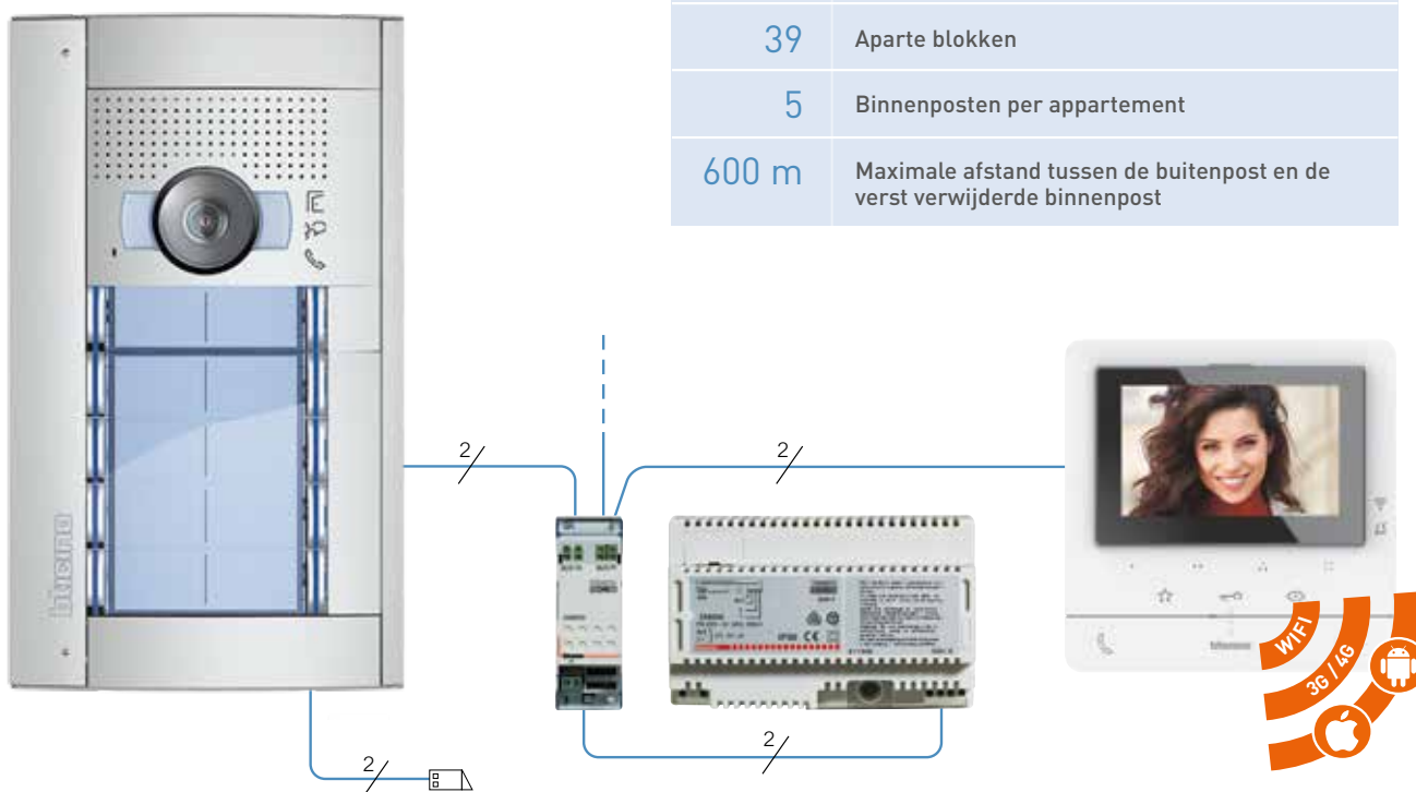
2 niet-gepolariseerde draden in heel de installatie
